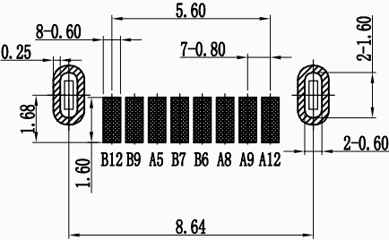
PCB板参考图
