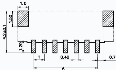
SH-AB PCB 寸法 PCB Layout
