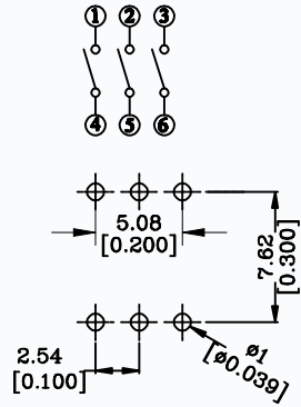
P.C.B. LAYOUT
