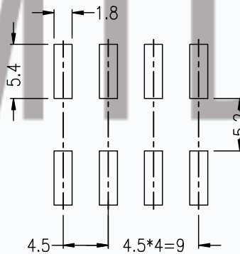
P.C.BOARD LAYOUT
