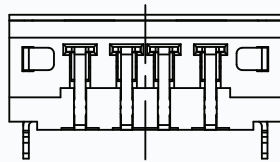
外壳铆合面视图
