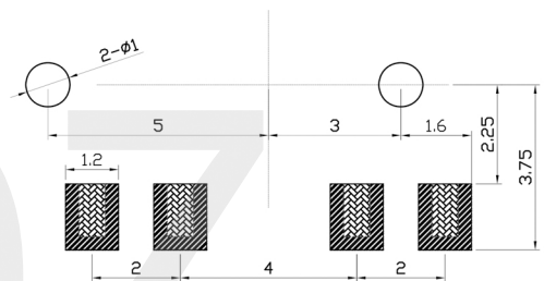
安装图 (PCB LAYOUT PLAN)
